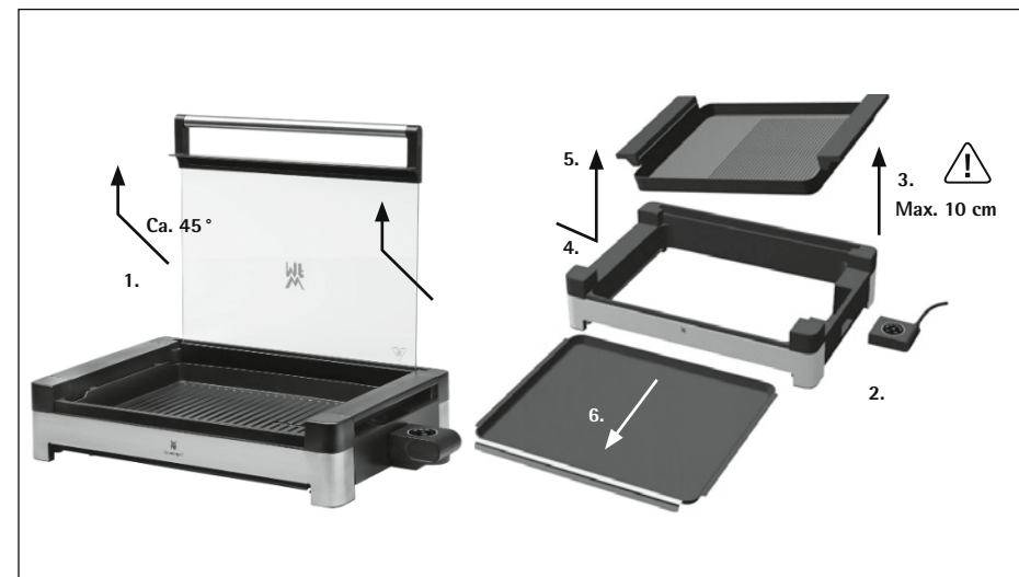
Фигура 2 - Демонтаж/Демонтаж
