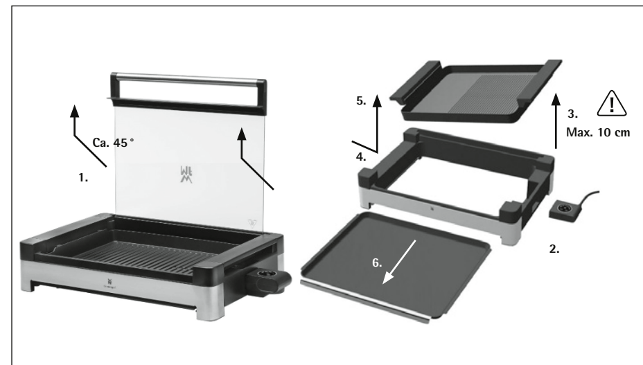
Рис. 2 – Демонтаж/разборка
