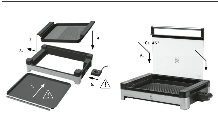
Abb. 1 - Zusammenbau/ Assembling
