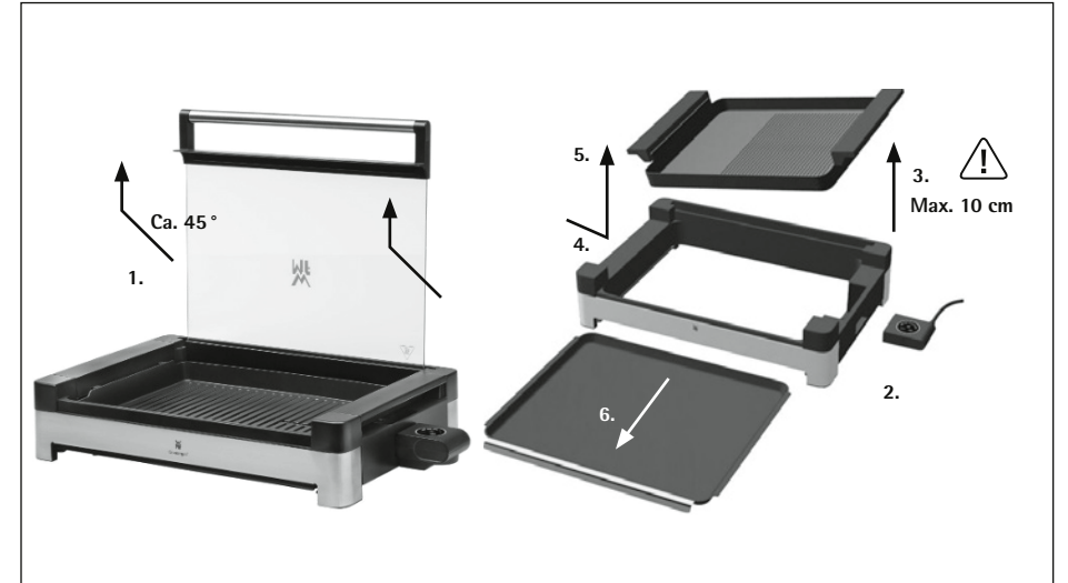
Şekil 2 - Demontaj / Sökme
