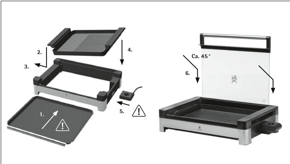
Şekil 1 - Zusammenbau/ Montaj
