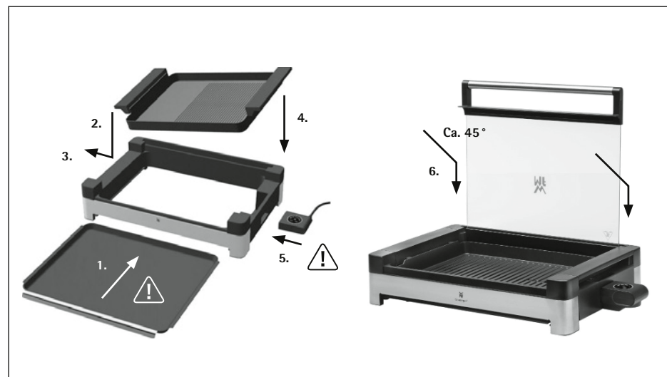
Fig. 1 - Zusammenbau/ Assembling
