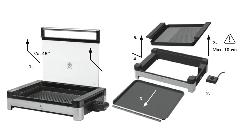
Kuva 2 - Demontage /Disassembling
